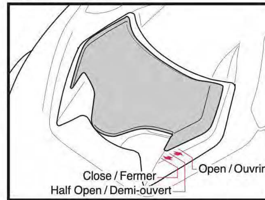
Upper Air Intake / Entrée d'air supérieure
