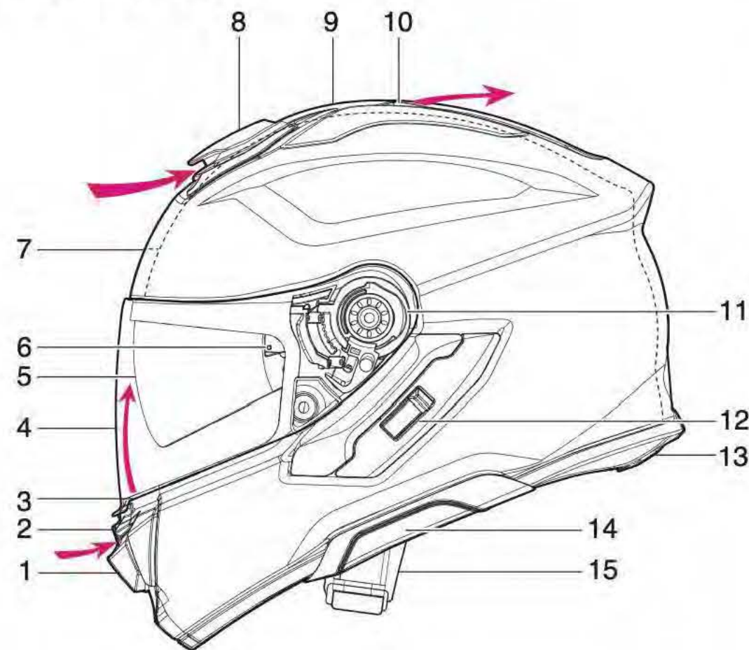
Upper Air Intake / Entrée d'air supérieure
